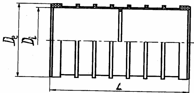
Рис. 2.1. Муфта для соединения труб «ЭЛЕКТРОКОР».
